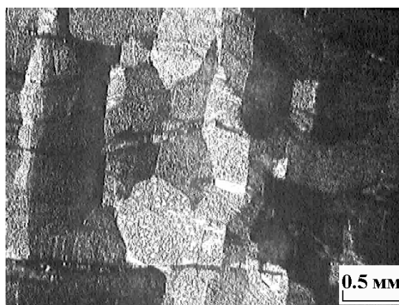
Рис. 9. Фотографія ділянок переорієнтації монокристулу NaCl, деформованого в процесі повзучості
