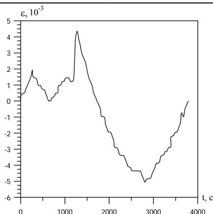
Рис. 1. Крива повзучості монокристала KCl після зменшення зовнішніх напружень від \sigma_1 = 0,8 МПа до \sigma_2 = 0,2 МПа, T = 650 °С
