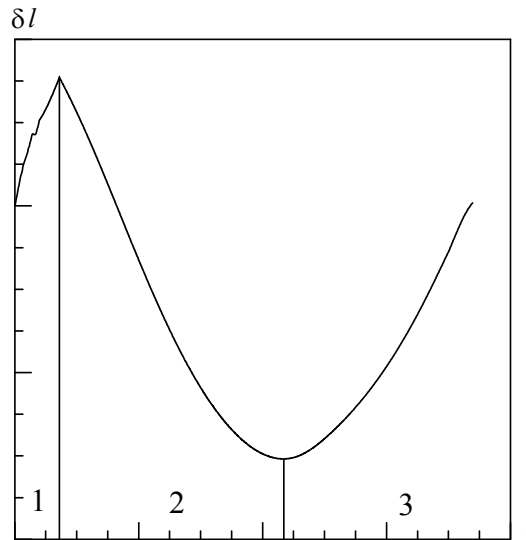
Рис. 2. Розрахована деформаційна крива при прориві дислокацій крізь дислокаційну межу
