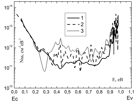
Рис. 3. Розподіл густини поверхневих станів у забороненій зоні кремнію на межі поділу Si-SiO 2 : 1 — вихідний монокристал кремнію; 2 — пластично деформований, тобто дислокаційний кремній; 3 — додатково окиснений дислокаційний кремній.
